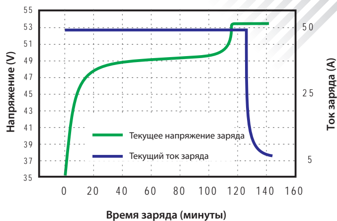
Характеристики заряда при 0.5C 25°C
