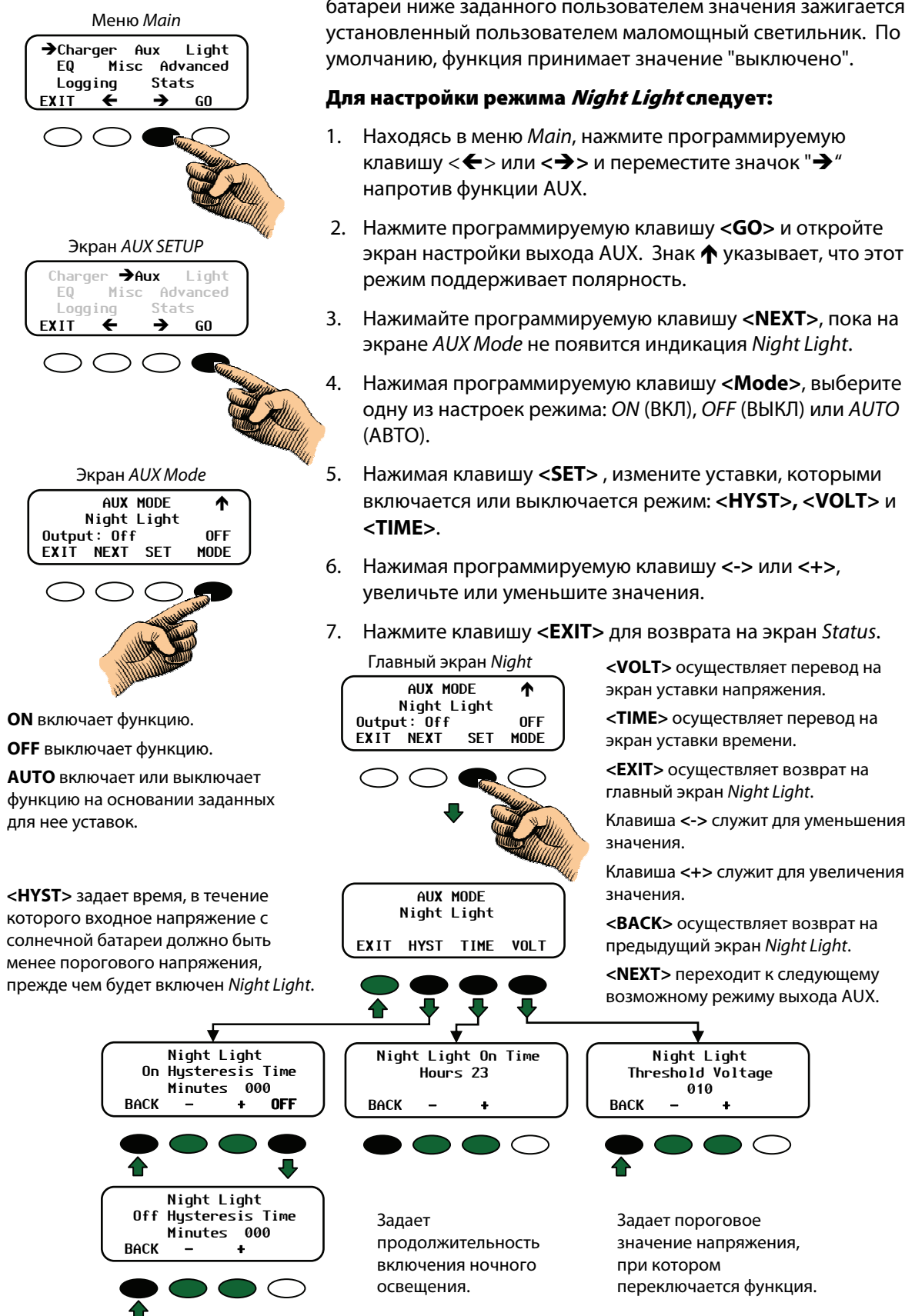
Рисунок 19 Настройка режима ночного освещения
