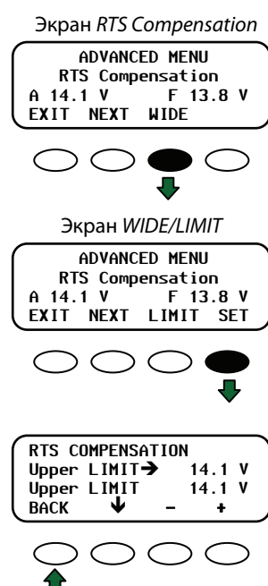
Рисунок 43 Компенсация RTS
