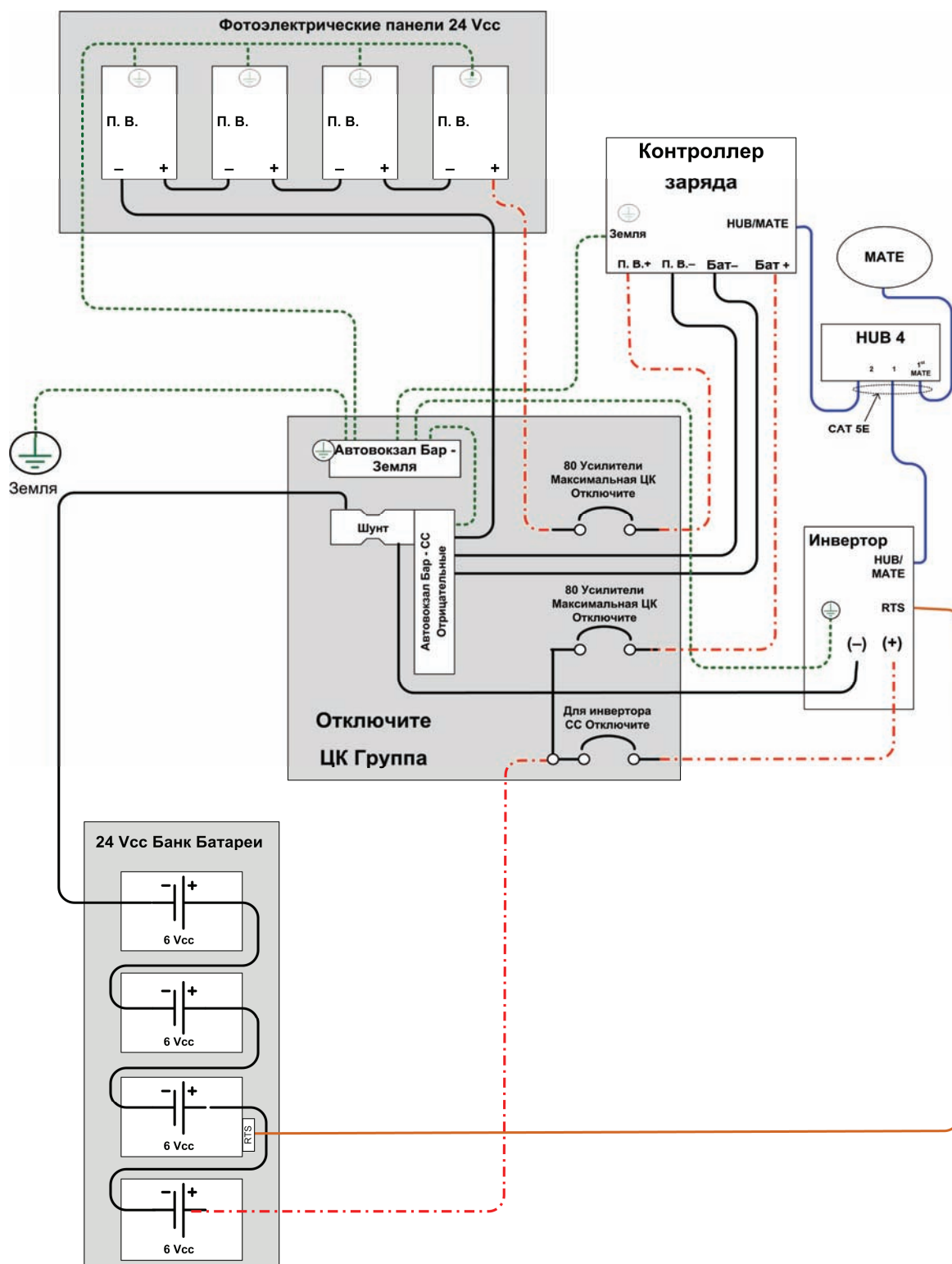
Рисунок 5 Принципиальная схема подключения одного контроллера зарядки к солнечной батарее напряжением 24 В
