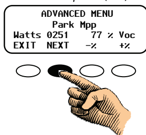
Рисунок 71 Настройка пределов диапазона поиска точки максимальной мощности для систем с микро-ГЭС или топливными элементами
