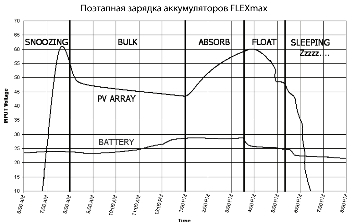
Рисунок 40 Поэтапная зарядка аккумуляторов FLEXmax
