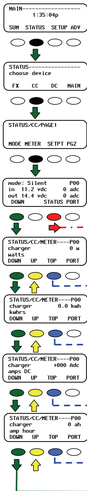
Рисунок 52 Экраны METER
