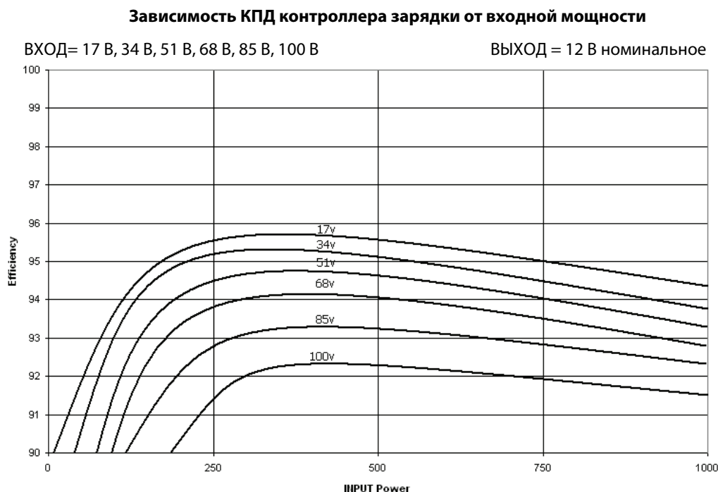
Рисунок 72 График КПД для системы с аккумуляторами напряжением 12 В
