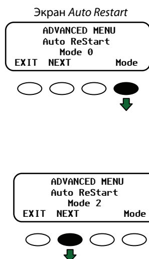
Рисунок 44 Автоматический перезапуск
