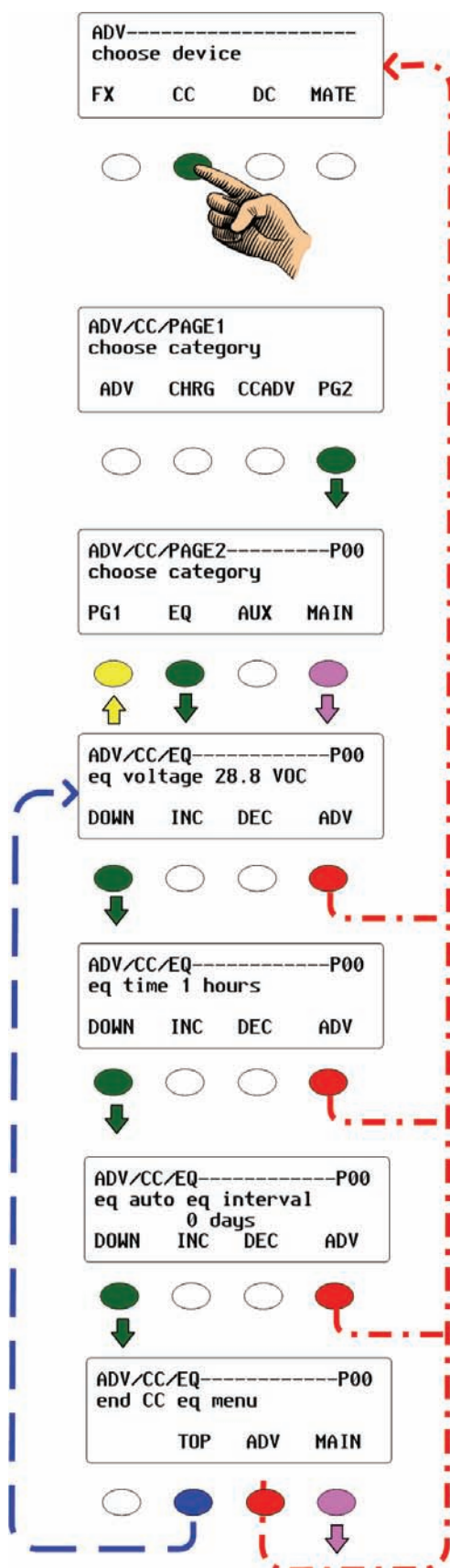
Рисунок 59 Меню ADV для функций зарядки EQ
